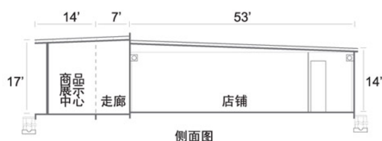
侧面图
